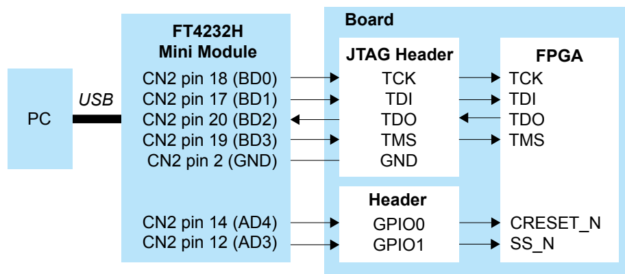
Figure 53: Connect FT4232H Mini Module to JTAG Pins plus CRESET_N and SS_N
